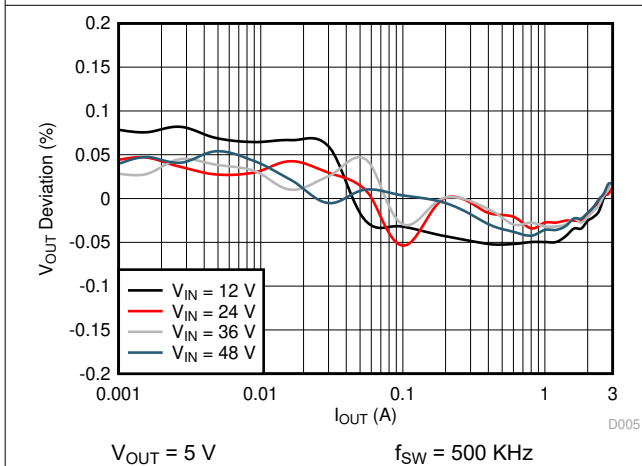
图 6-5. Load Regulation
