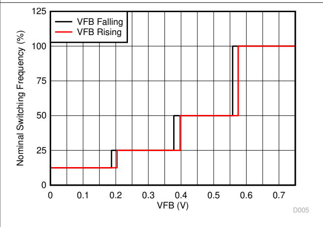
图 6-6. Frequency vs. VFB
